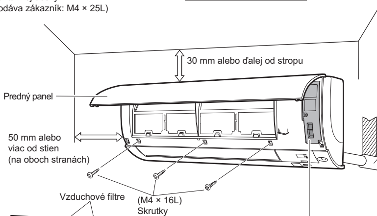
Upevňovacia skrutka montážnej dosky (dodáva zákazník: M4 × 25L)
